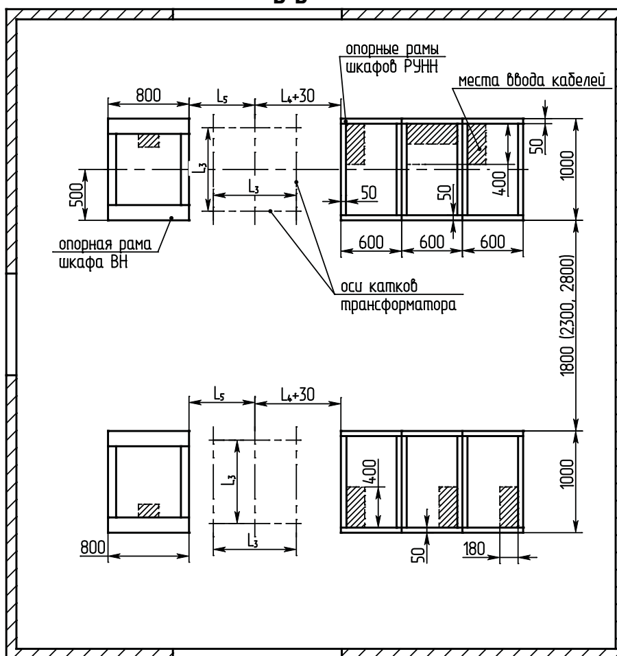
Габаритные и установочные размеры 2КТПСП
