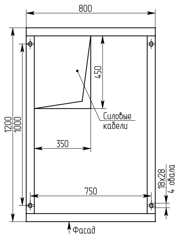
Рис. Г.14. шкаф 4ШНХХ-13 с расположением силовых ячеек на II секцию подстанции
