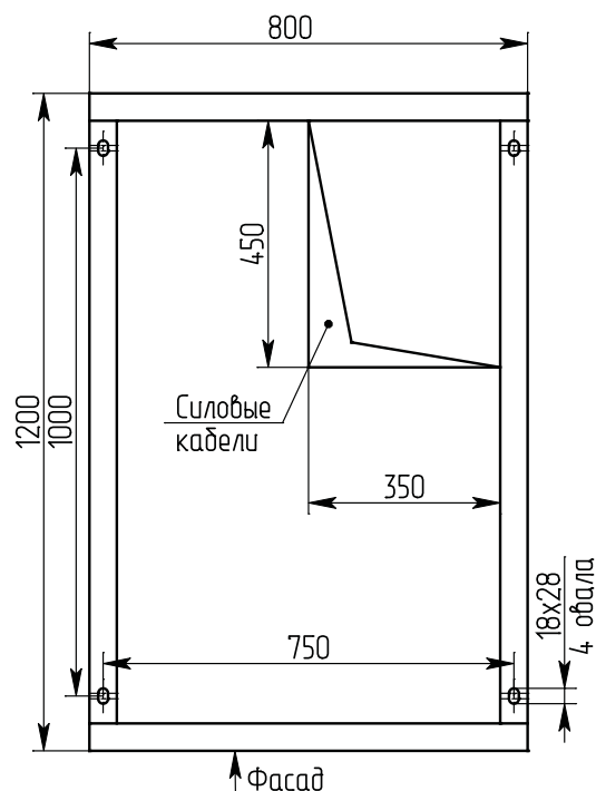
Рис. Г.16. шкаф 4ШНХХ-13 с расположением силовых ячеек на I секцию подстанции
