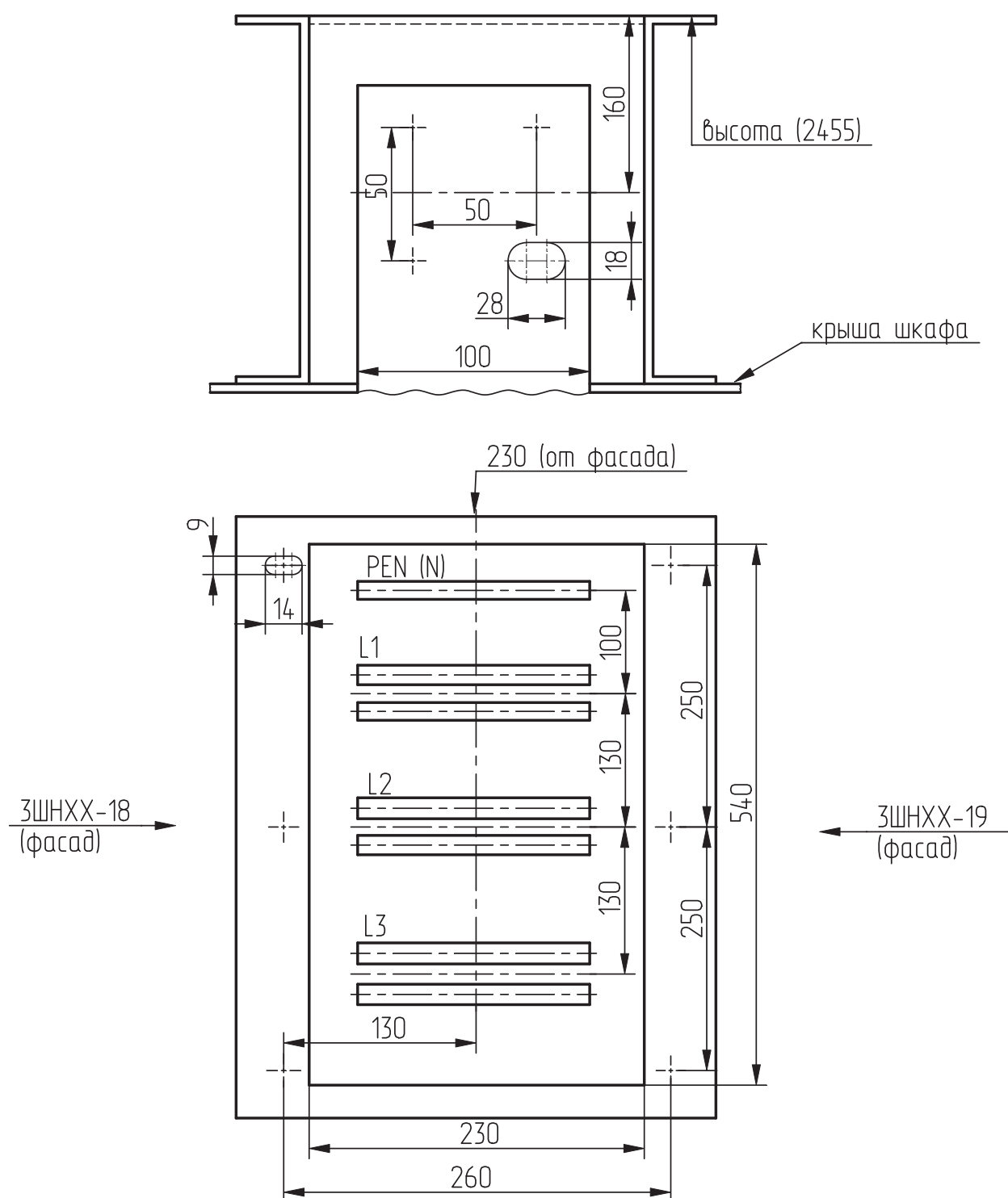
Рис. Д.2. Присоединительные размеры для установки шинопровода на номинальный ток 2500 А
