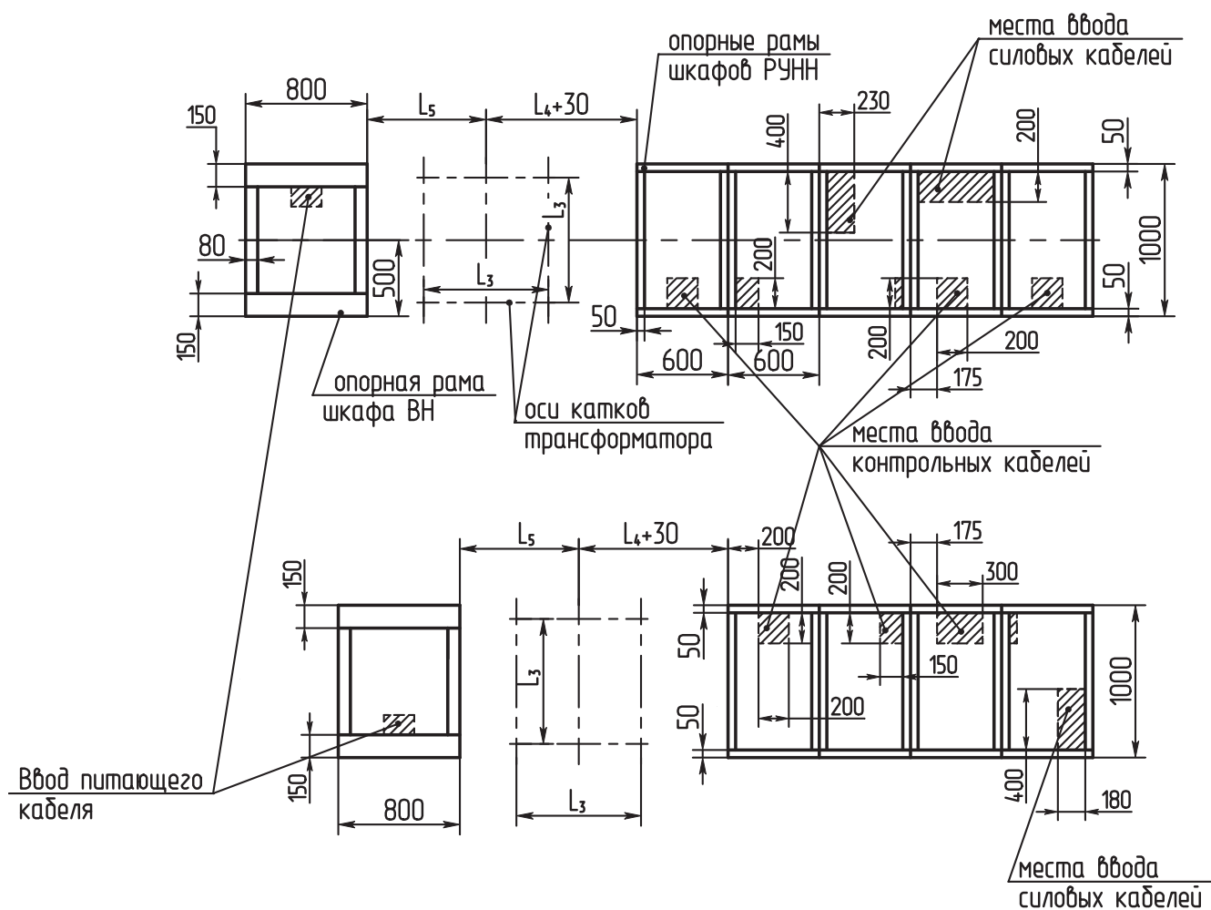
Габаритные и установочные размеры 2КТПЦ
